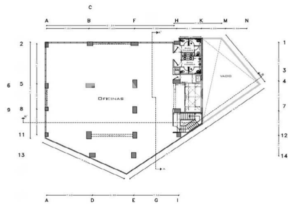
NIVEL 9 AL 18 PH — OFICINAS TIPO
